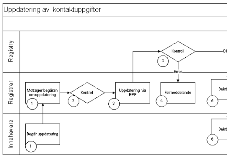
Figur 3: Flödesschema - Uppdatering av kontaktuppgifter
