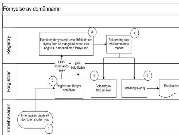
Figur 2: Flödesschema - Förnyelse av domännamn
