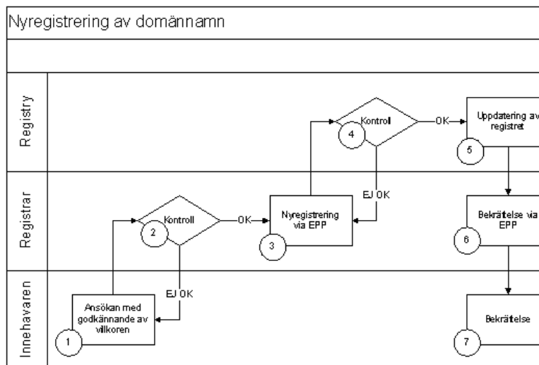
Figur 1: Flödesschema - Nyregistrering av domännamn
