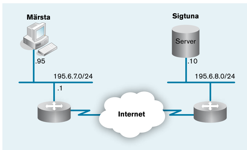
Nätskiss hur IP-klienten i Märsta når servern i Sigtuna
